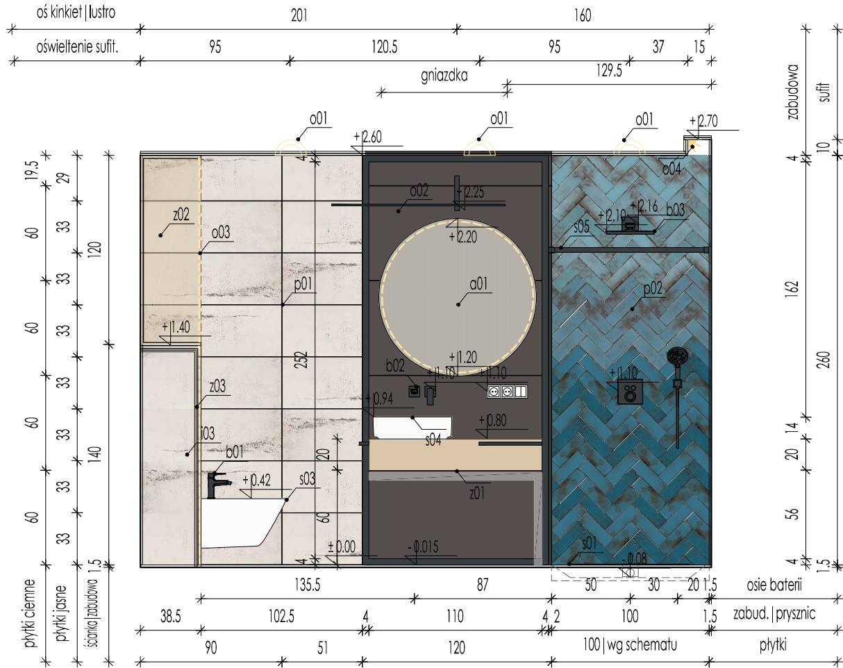
WIDOK A-A
