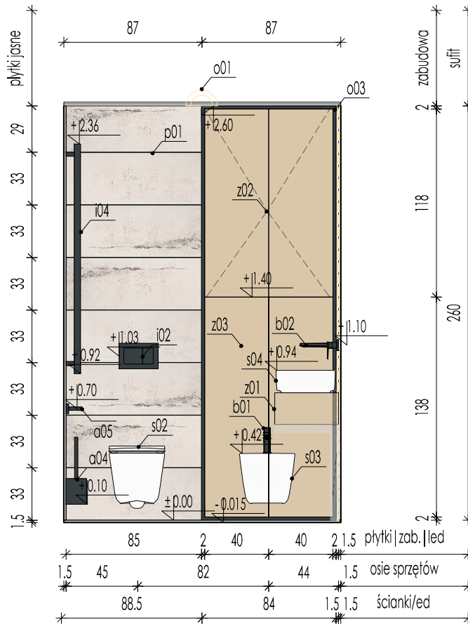
WIDOK D-D
